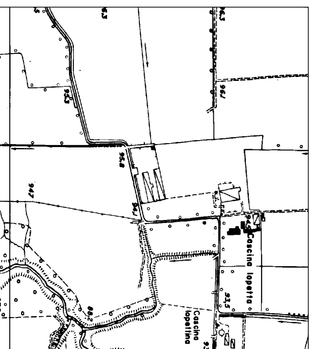
Stralciato di carta tecnica regionale (volo 1994)
